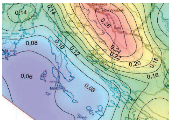
Slika 2. Vršna ubrzanja tla uzrokovana potresima za područje Grada Malog Lošinja za povratni period 475 godina
