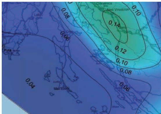
Slika 3. Vršna ubrzanja tla uzrokovana potresima za područje Grada Malog Lošinja za povratni period 95 godina
