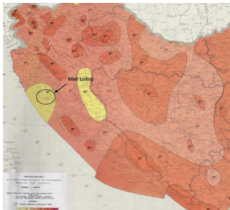
Slika 1. Seizmološka karta za povratni period od 500 godina
